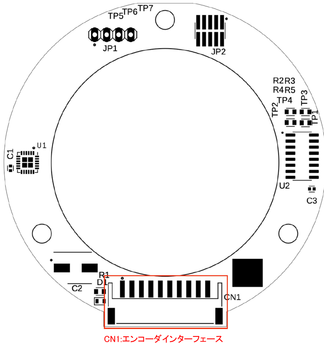
Fig.2 コネクタ位置
