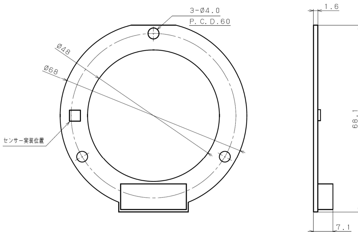
Fig.1 基板外形
